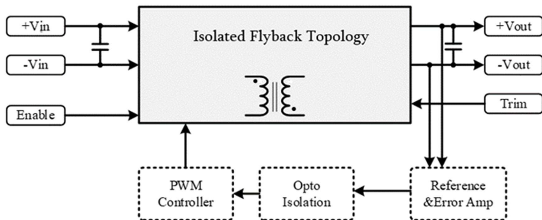
ESBS 单路电路图
