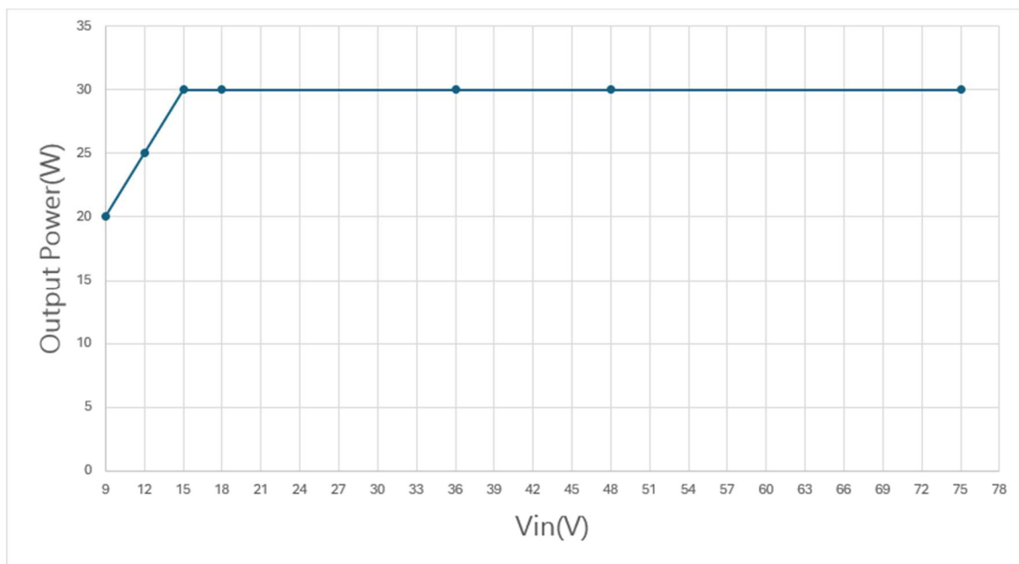
输出额定功率 VS 输入电压
