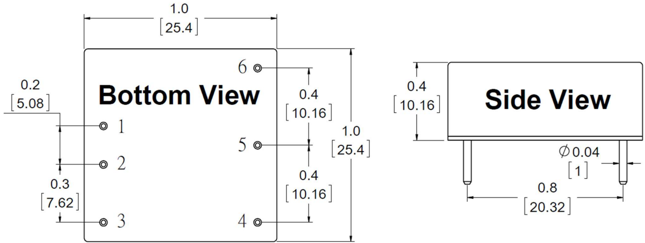
尺寸图 - F 平壳
