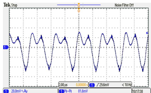
图 8: 出输出电压纹波与噪声(满载). (典型输入, 于输出端加 1μF MLCC 陶瓷电容))
