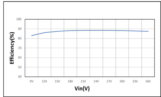
图 2: 效率值 VS 输入电压(满载)
