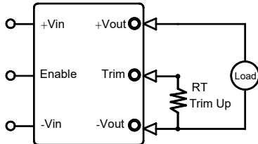
图 1. 电阻调整输出电压示意图(上调)
